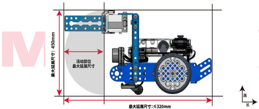
图 5.1-1 最大延伸尺寸-侧视图
