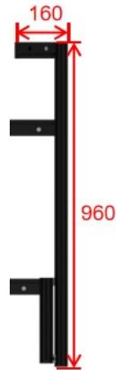
图 4.2-18 旗帜悬挂尺寸图（正视图）
