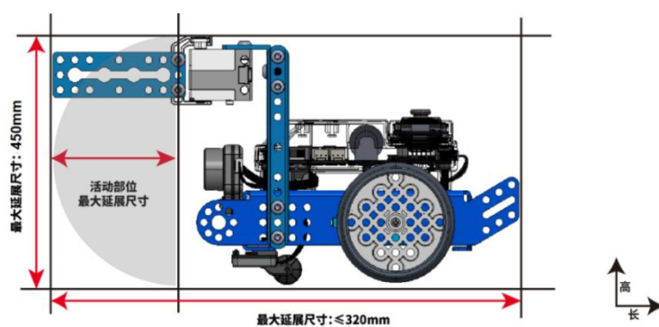
图 5.1-1 最大延伸尺寸-侧视图
