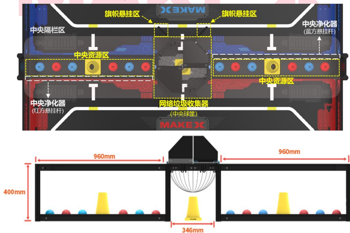
图 4.2-6 中央隔栏区域示意图
