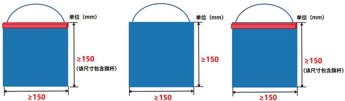
图 4.3-3 净网旗帜示意图
