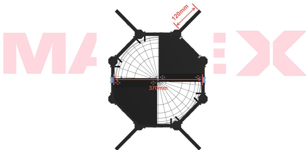
图 4.2-11 旗帜悬挂区尺寸图
