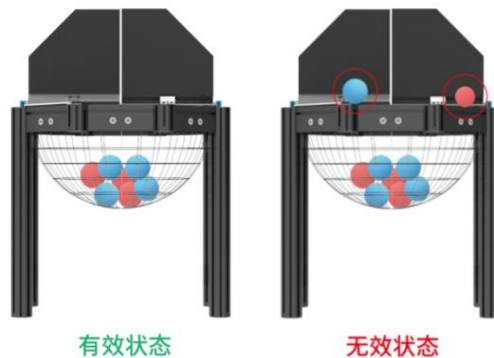
图 4.4-1 球类得分状态判定
