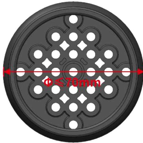
图 5.1-3 车轮尺寸图
