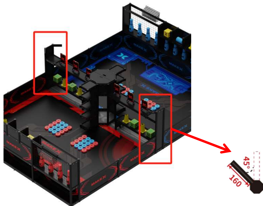
图 4.2-17 旗帜悬挂区示意图（侧视图）
