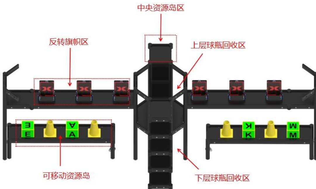
图 4.2-5 中央资源区示意图（轴视图）
