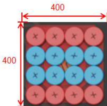
图 4.2-19 红方圆饼摆放示意图（俯视图）
