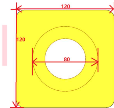
图 4.3-8 锥桶示意图（仰视图）
