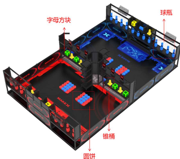
图 4.3-1 场地道具摆放示意图
