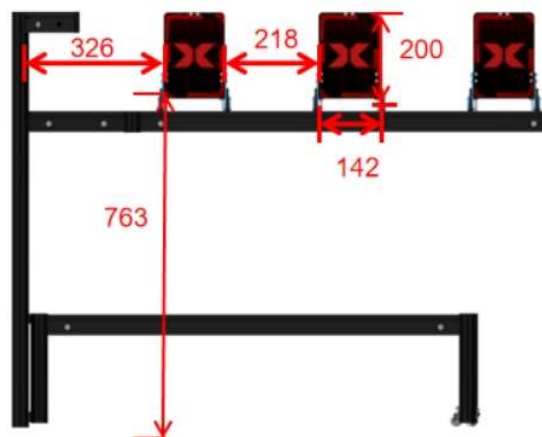
图 4.2-8 反转旗帜区示意图（正视图）
